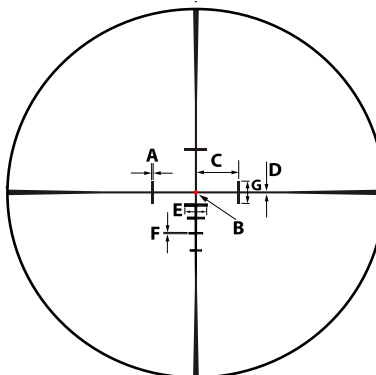
3TR/P3TR RETICLE SUBTENSION
