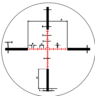
G28 MIL DOT RETICLE SUBTENSION
